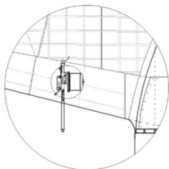
Montage de la mitrailleuse dans l'aile
