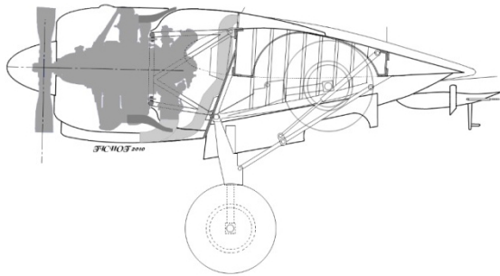
Coupe du fuselage moteur
